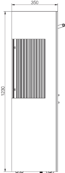
Technische Zeichnung RITON BIOETHANOL
